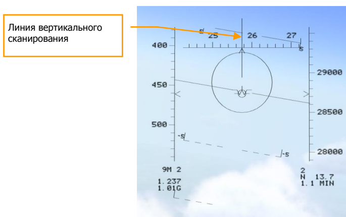
4-32: Режим вертикального сканирования (VS)
