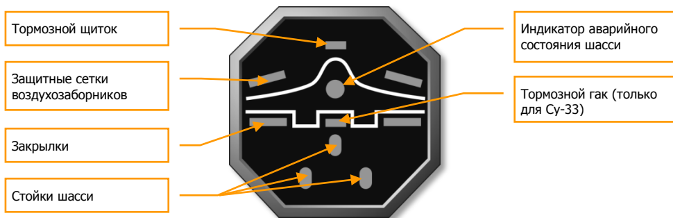
3-5: Пилотажно-посадочный индикатор
