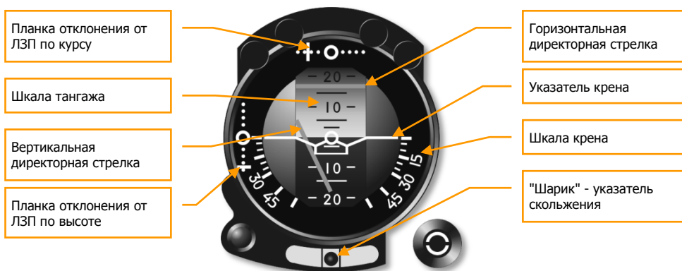
3-7: Командно-пилотажный прибор (КПП)
