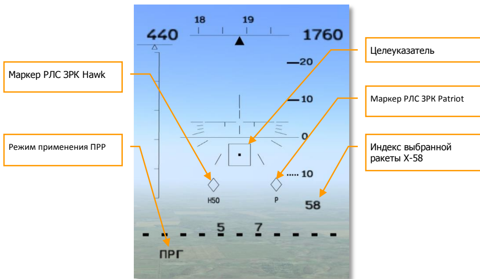
3-67: Вид ИЛС в режиме целеуказания ПРП
