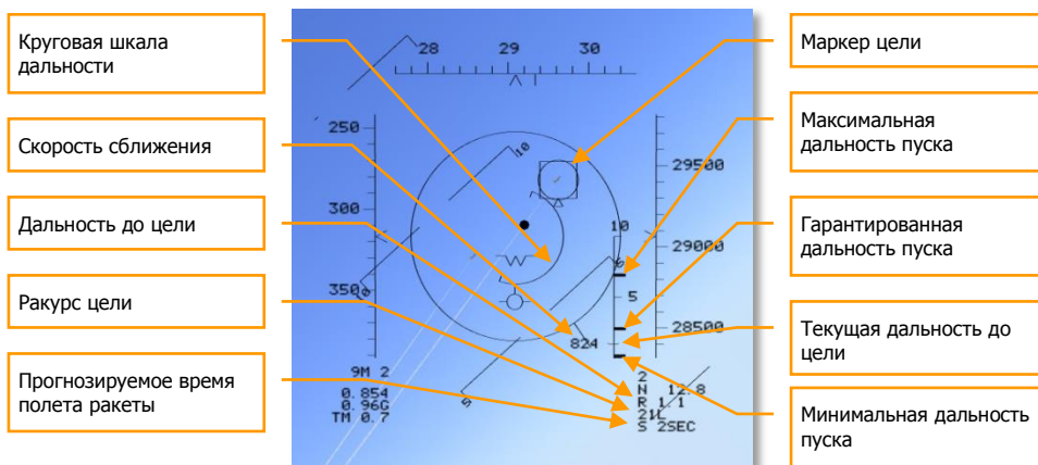
4-26: Режим STT. Применение ракет ближнего боя при захвате цели РЛС на дальности менее 12 000 футов
