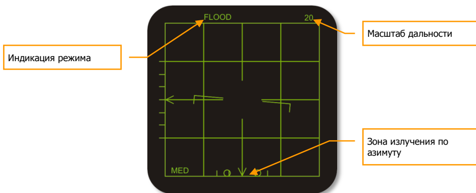
4-40: Режим Flood
