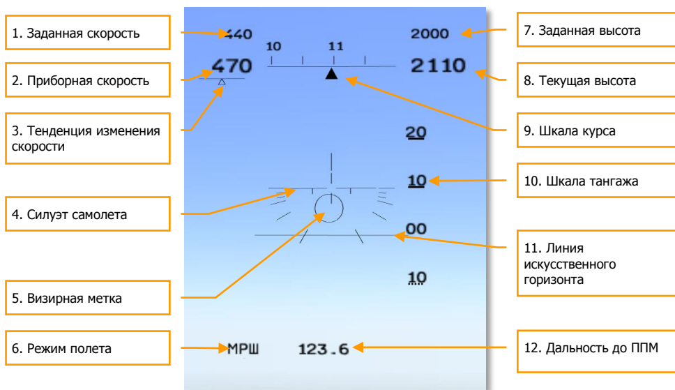
3-18: Базовая символика на ИЛС МиГ-29
