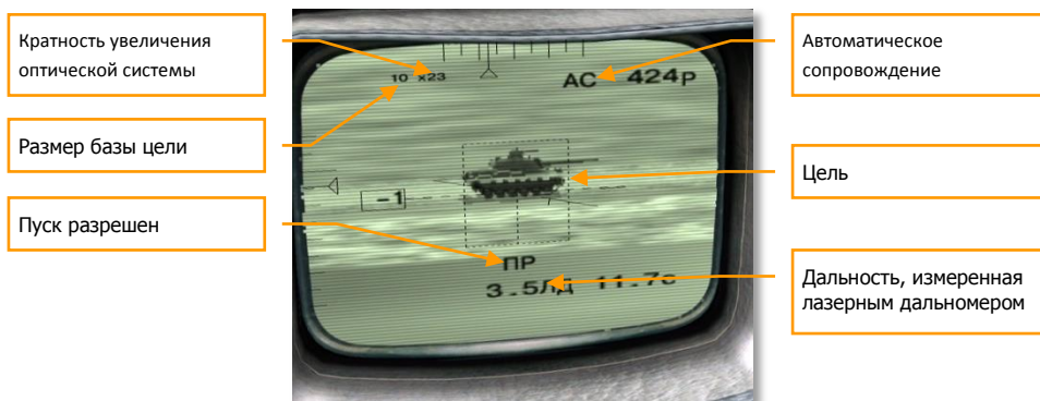
З-66: Вид ТВ-индикатора ИТ-23М при автоматическом сопровождении цели прицельным комплексом Шквал с включенным лазерным дальномером
