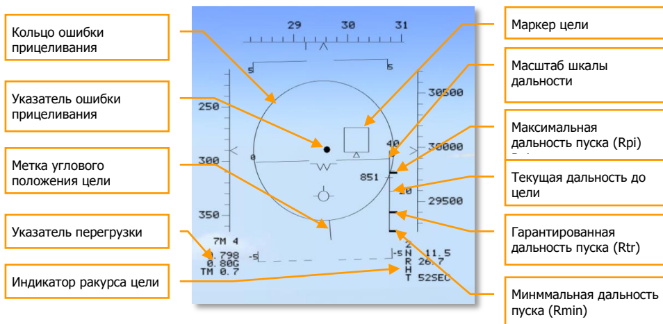
4-28: Режим STT. Применение ракет AIM-7M в дальнем ракетном бою
