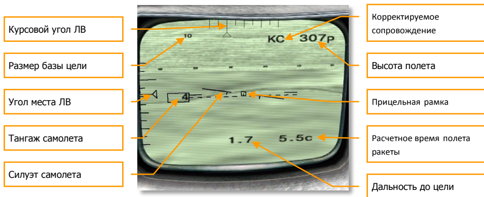
3-65: Вид ТВ-индикатора ИТ-23М при поиске цели с включенным прицельным комплексом Шквал
